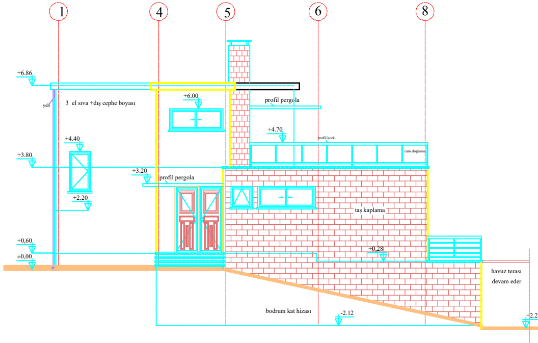
ÖN CEPHE ÖLÇEK:1/50
