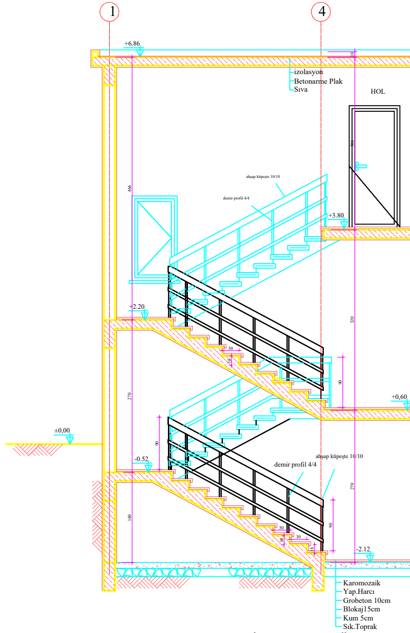
A-A KESİT DETAYI ÖLÇEK:1/20
