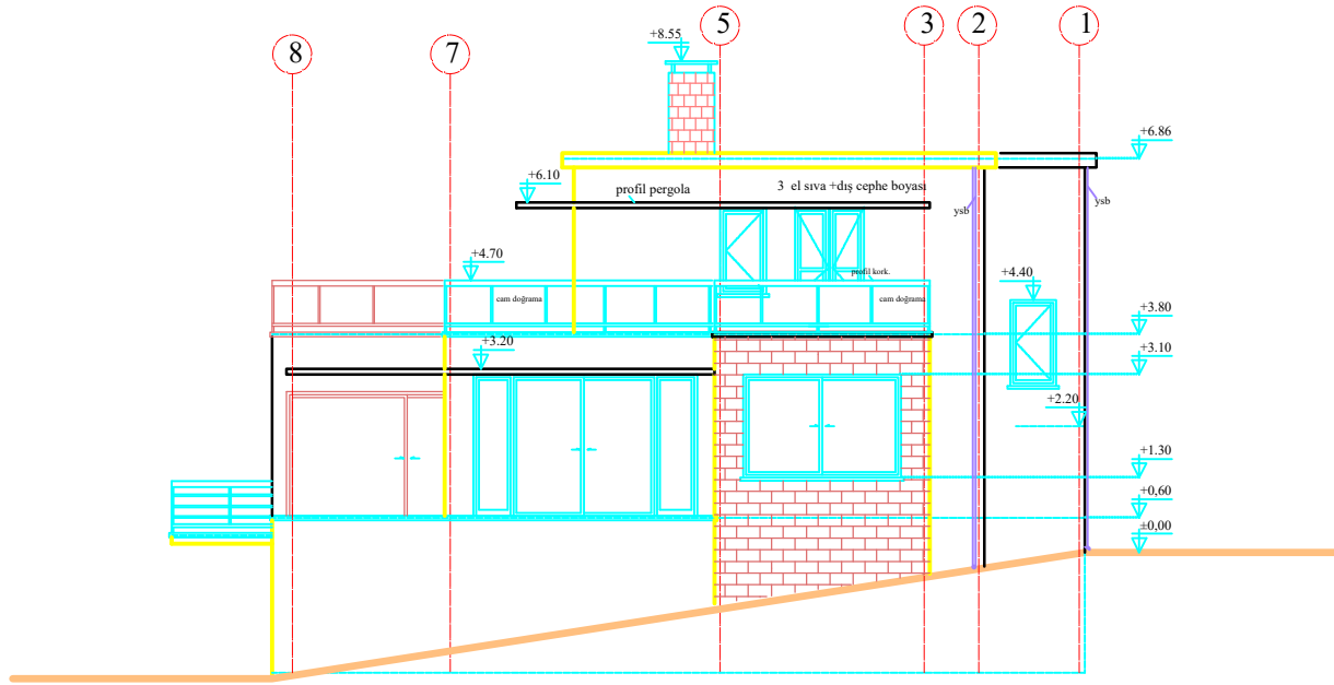
ARKA CEPHE ÖLÇEK:1/50
